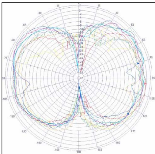
Rad. Pattern
